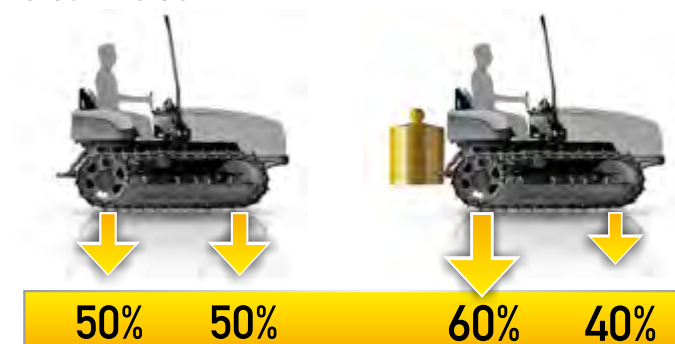
ORUGA TRADICIONAL
