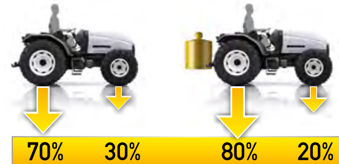
TRACTOR TRADICIONAL
